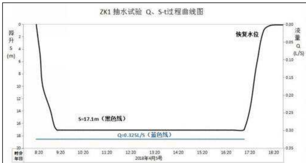
图 5.2-11 抽水试验 Q、S-t 过程曲线图
