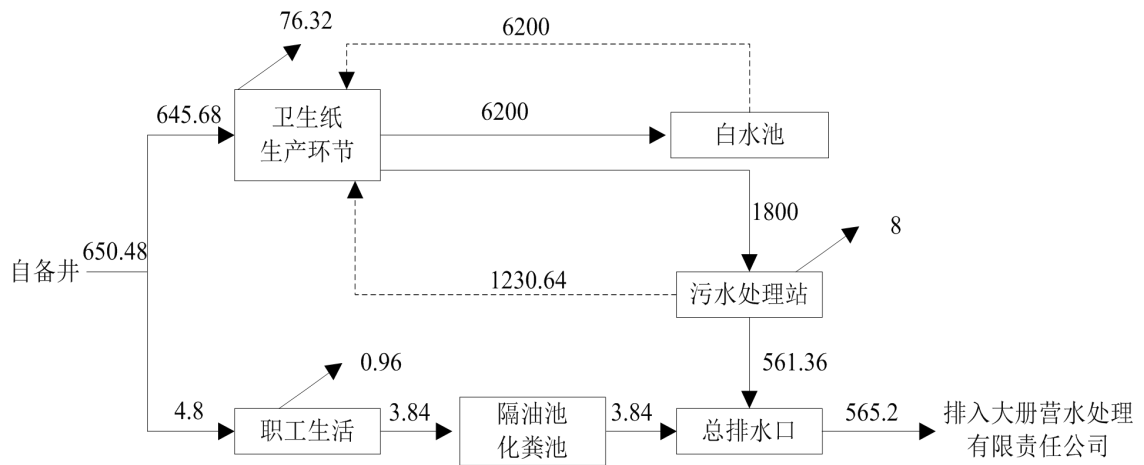
图 3.1—3 水平衡图 (m 3 /d)
