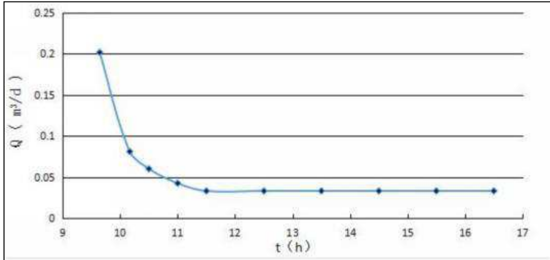
图 5.2-10 SK2 渗水试验 Q-t 历时曲线图
