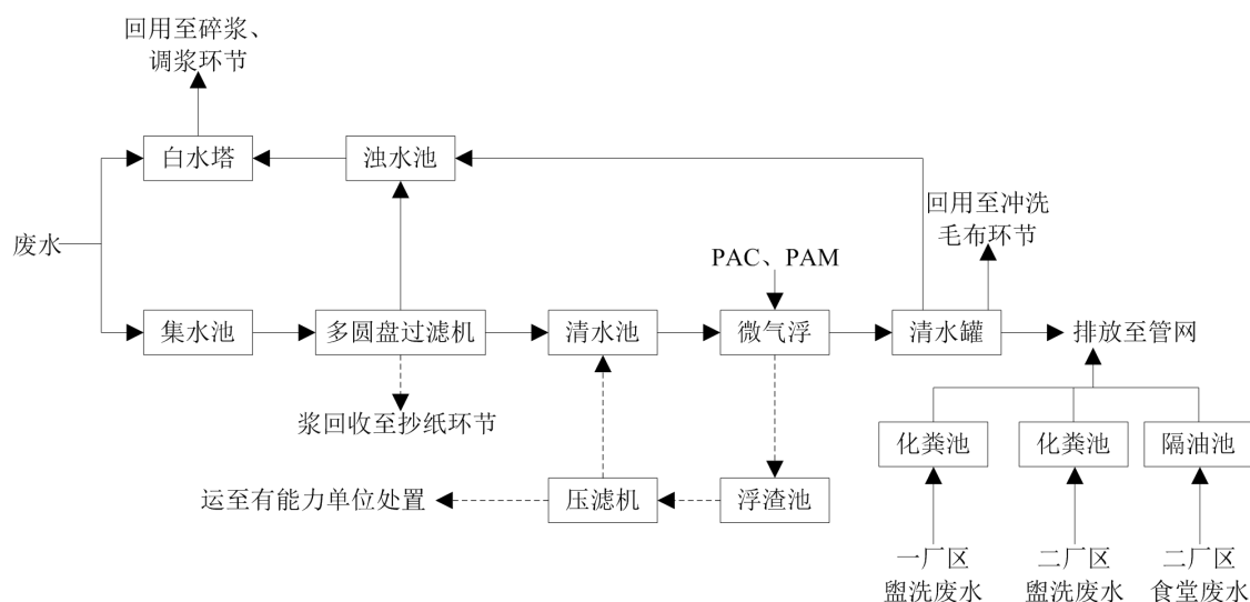
图 6.2-1 改扩建后污水处理工艺流程图
