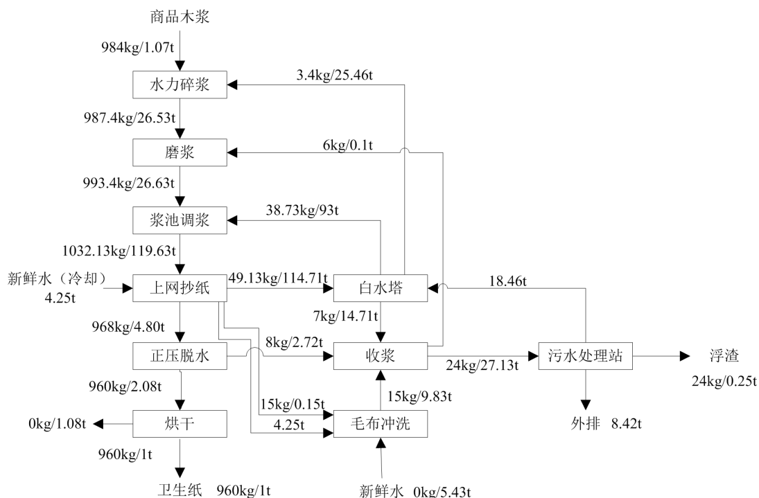
图 3.1-4 现有项目浆水平衡图 (绝干浆量 (kg) / 浆水总量 (t))
