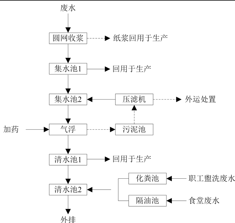
图 3.1-5 现有项目废水处理工艺流程图
