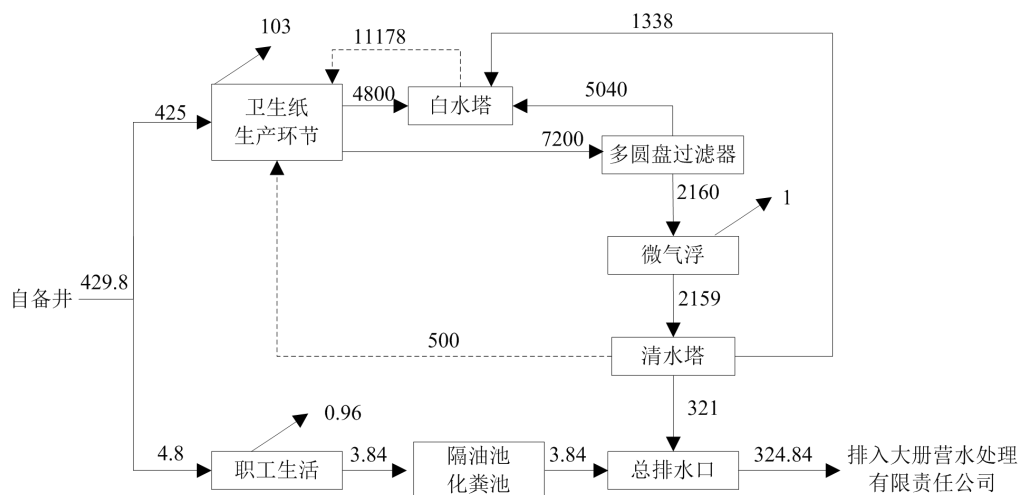
图 3.4-2 水平衡图 (m 3 /d)
