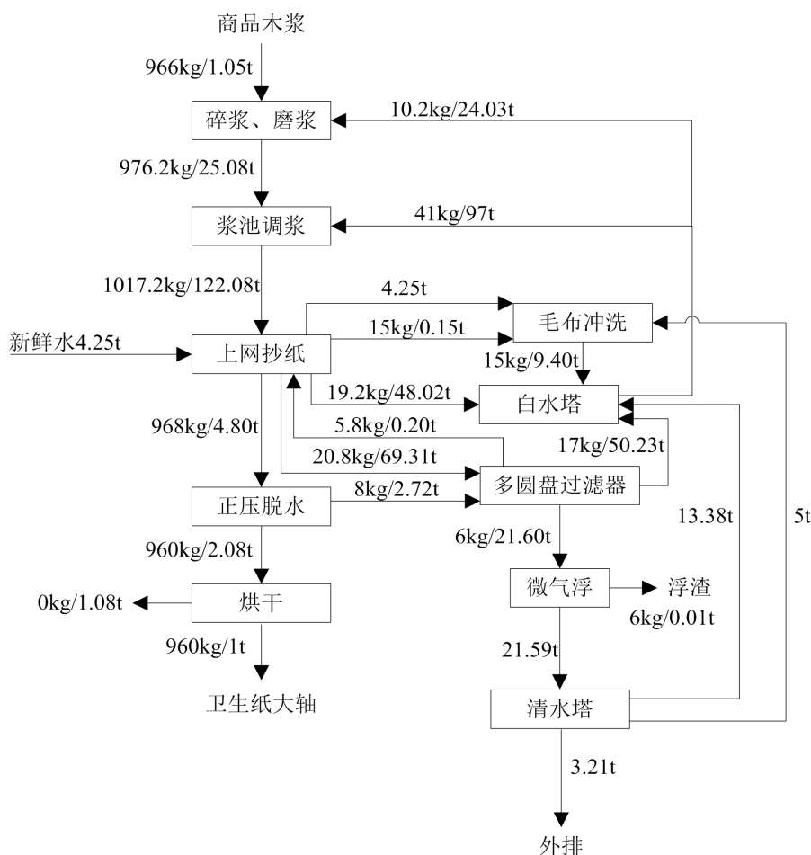
图 3.4-3 改扩建后全厂浆水平衡图（绝干浆量（kg）/浆水总量（t））
