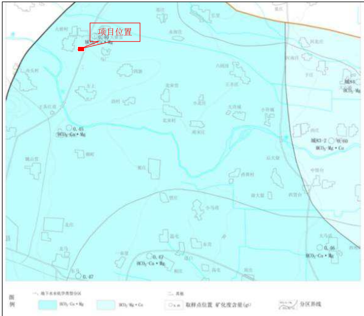
图 5.2-5 区域地下水水化学类型分布图
